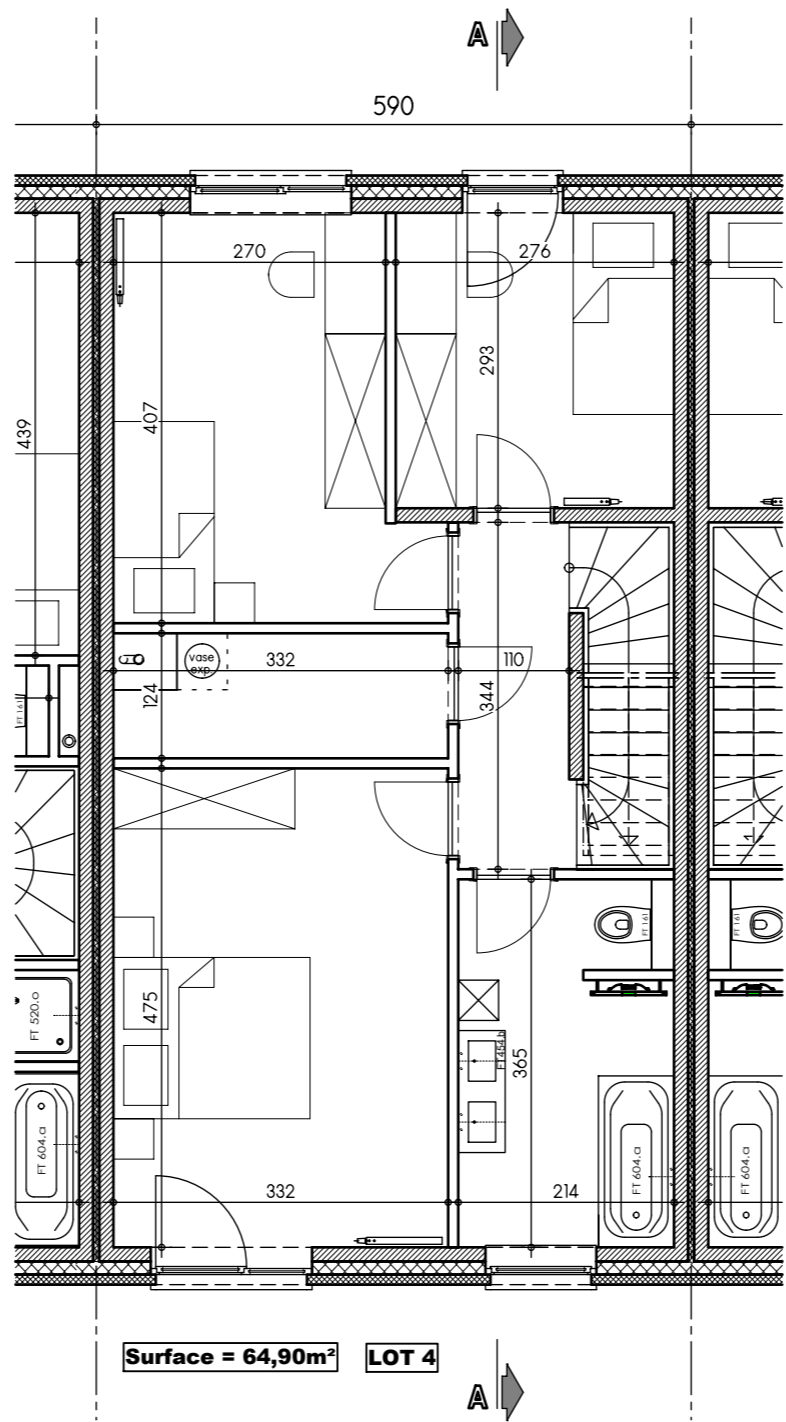
PLAN ETAGE
