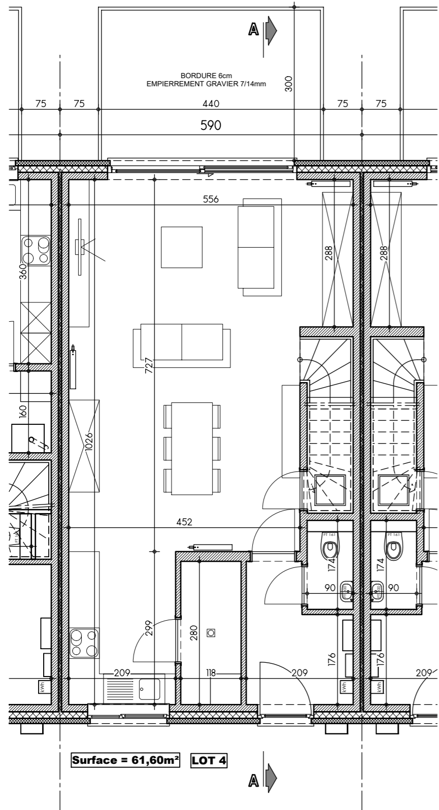
PLAN REZ-DE-CHAUSSEE
